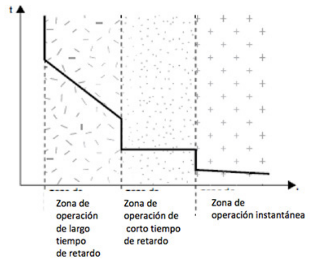
ZONA DE ACTIVACIÓN DE UN DISYUNTOR ELECTRÓNICO
